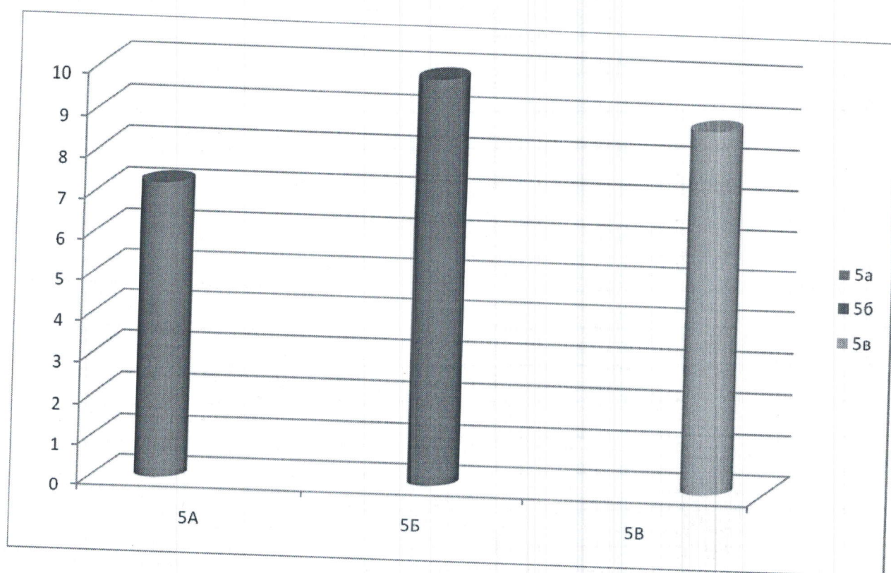
Гистограмма данных:
