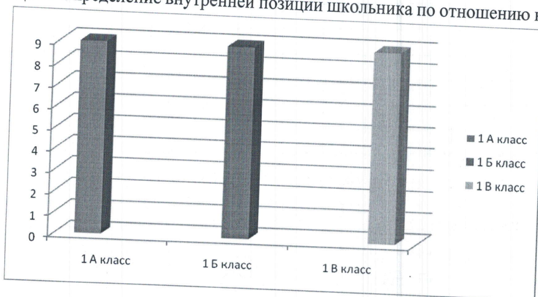
Гистограмма данных
